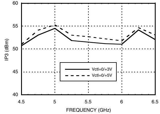
Input IP3 *
